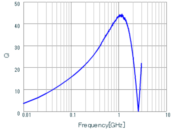
LQG15WH30NH02 Q.
