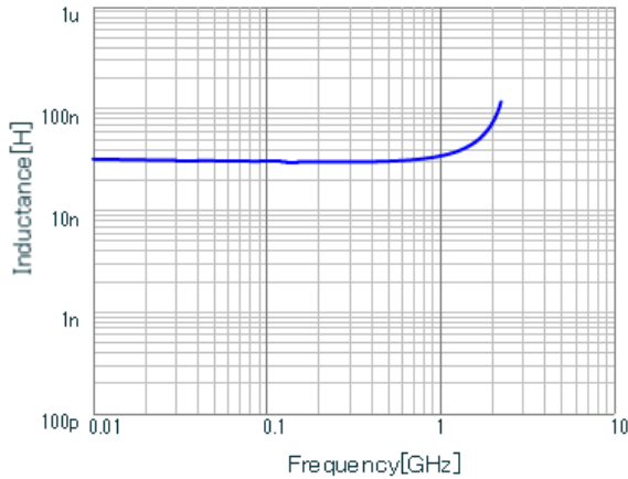
LQG15WH30NH02 L.
