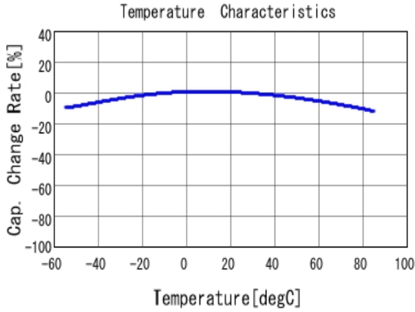
■ GRM033R61C224KE14 C-Temp. capchange, DCO. 0V, ACO. 2Vrm
