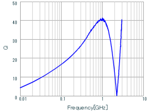
LQG15WZ36NG02 Q.
