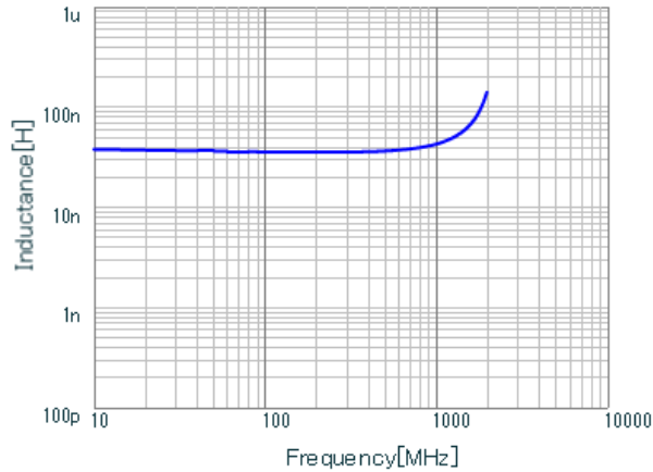
LQG15WZ36NG02 L.
