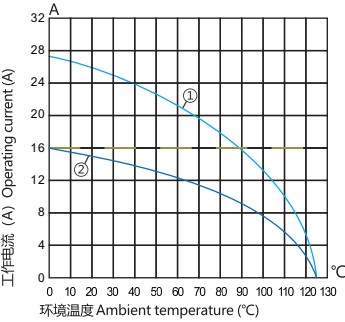
① 2.5mm² ② 1.5mm²
